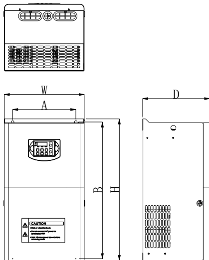
图 2-4. 22~160KW 变频器外型尺寸及安装尺寸示意图
