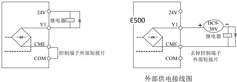
图3-7. 数字输出端子Y1接线示意图
