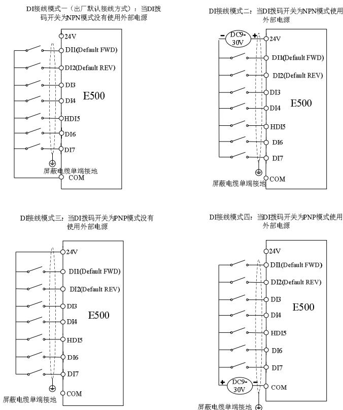
图3-6. 四种不同模式下数字输入端子接线图
