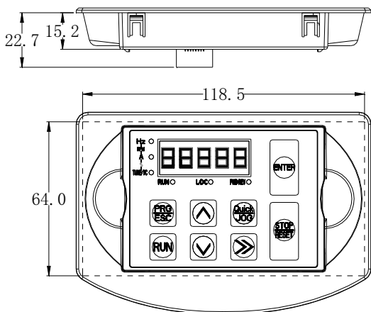
图 2-5 E500 大键盘 1 带托盘安装尺寸图
