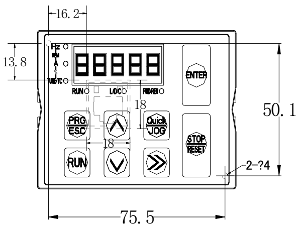
图 2-6 E500 大键盘 1 不带托盘安装尺寸图
