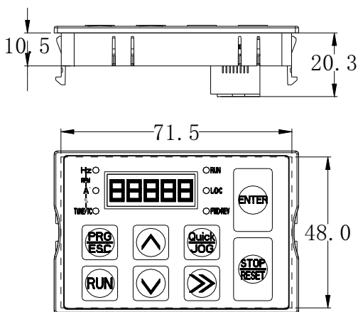
图 2-7 E500 小键盘 1 安装尺寸图
